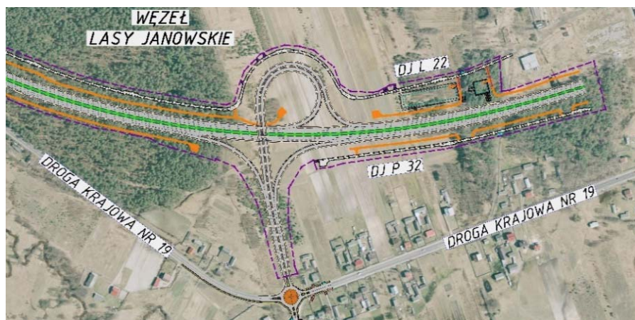
Rysunek 3. Prezentacja geometrii węzła Łasy Janowskie
