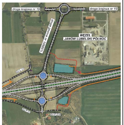
Rysunek 3. Prezentacja geometrii węzła Janów Lubelski Północ
