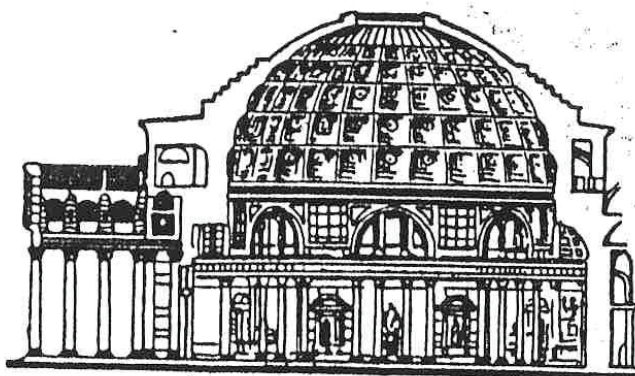
Przekrój Panteonu
